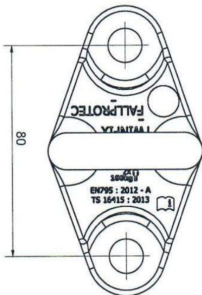
ankerpunt TwinFix
