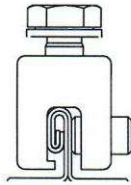
Principe knelbevestiging op de staande naad
